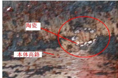
附图-1-4 高 Cr 陶瓷复合板锤局部解剖图
