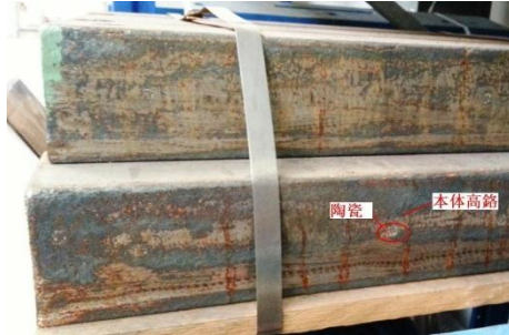
附图-1-3 高 Cr 陶瓷复合板锤外观图
